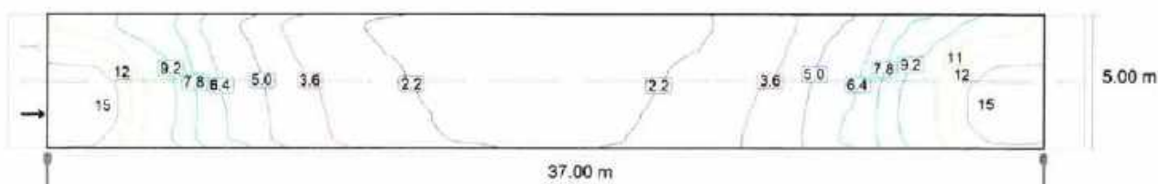
Valoarea de întreținere, intensitatea de iluminare orizontală [lx] (Linii Isolux)
